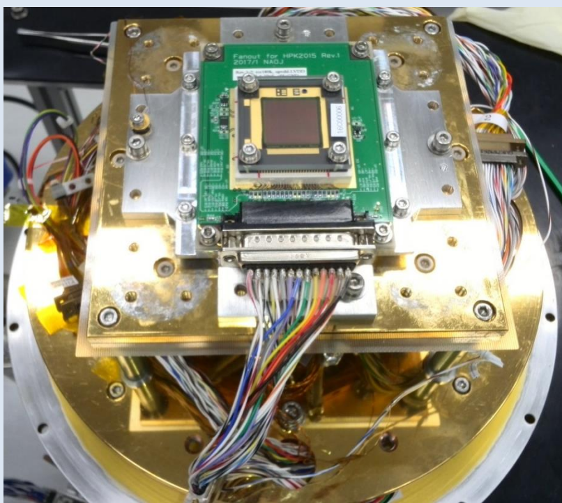
図3: 1.3k×1.3k InGaAs検出器
