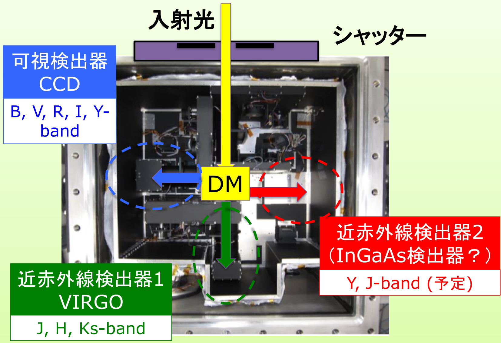
図2: HONIRを上から見た図
