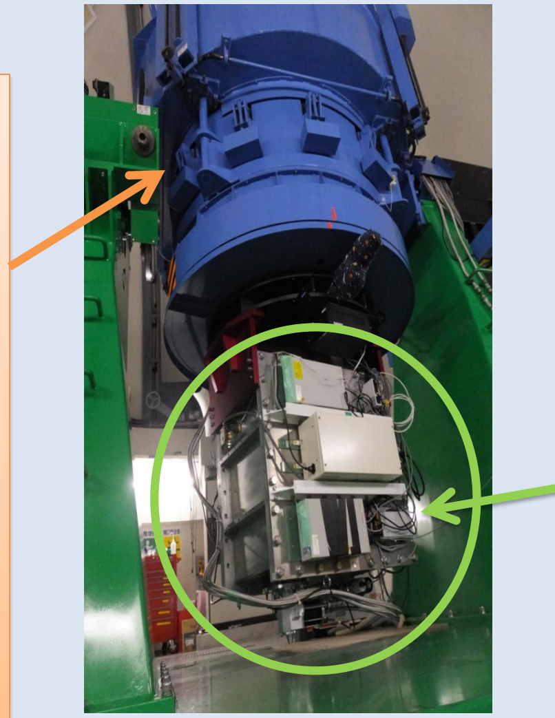
図1: かなた望遠鏡とHONIR
