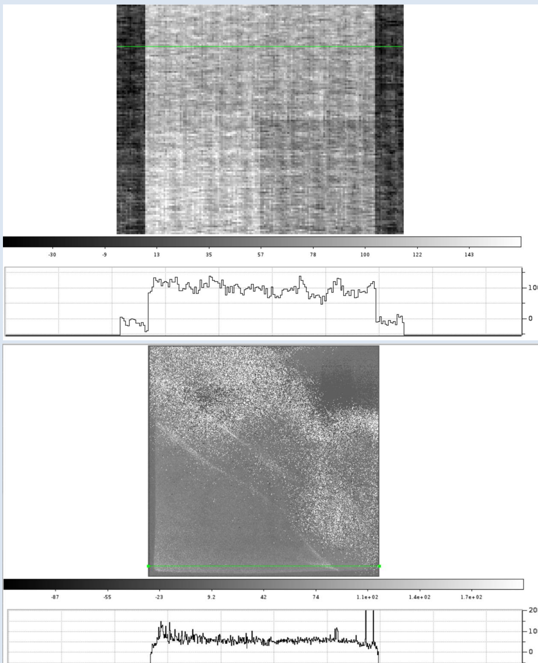
図8: dark画像のカウンターの横断面図 上→128pix素子 50s積分 左右の黒いピクセルはreferenceピクセル 下→1.3k素子 102s積分
