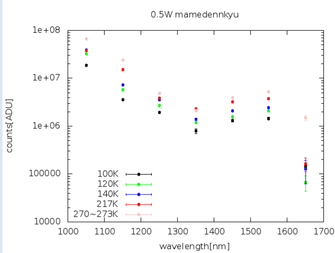
図4: 0.5W豆電球を用いた波長-信号強度のグラフ
